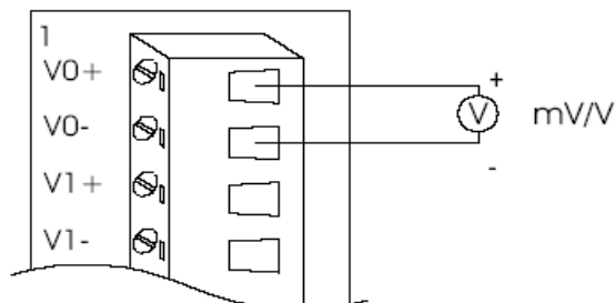
Figure 1.9 Millivolt and Volt Input
