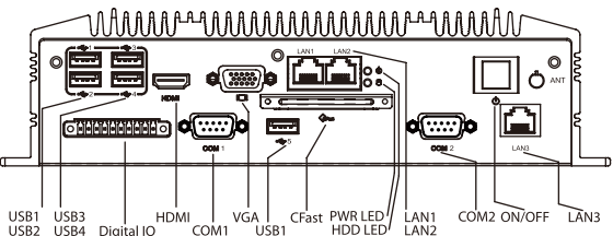
前面板外置I/O视图
