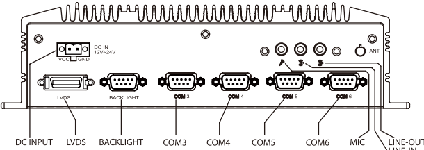
后面板外置I/O视图
