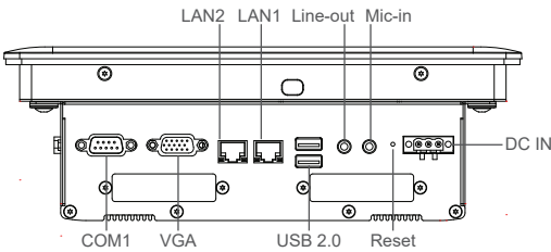
Right I/O
