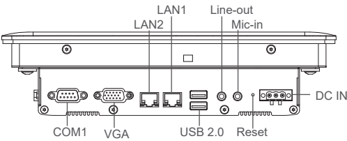
Right I/O
