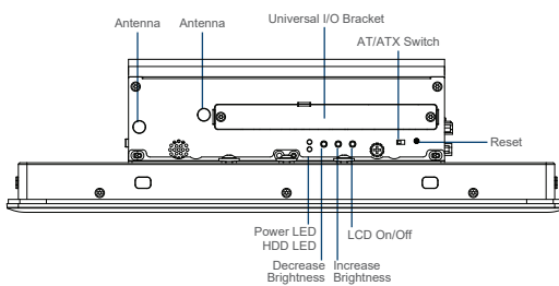
Left I/O
